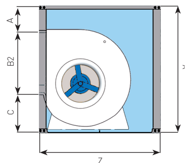
VISTA LATERALE
